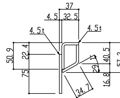
嵩上げ材詳細図
