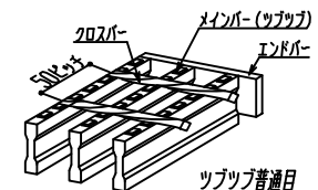
嵩上げ材詳細図
